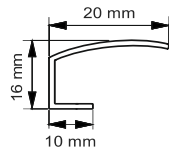
Standard Führungsschiene
